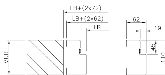
Typ D, EI 2 60, slagdörr
